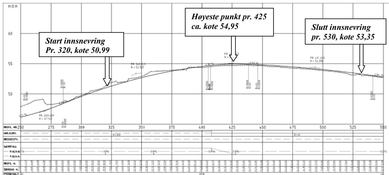
Lengdeprofil for alle alternativene på strekningen kryss med «Prestdalsveien» - kryss Grønnslettveien
